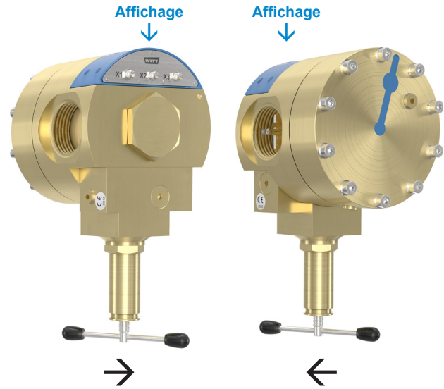
Position d'installation du 757LE/S Smart
