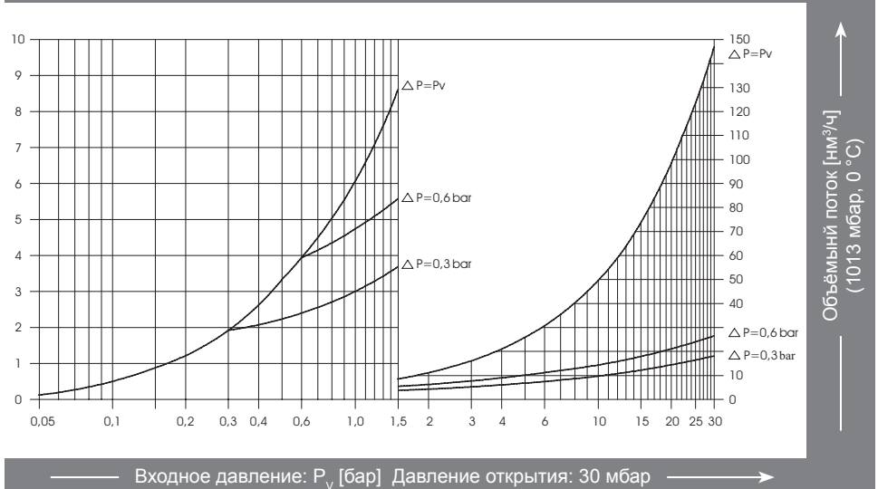
Диаграмма пропускной способности (воздух, 20 °С)
