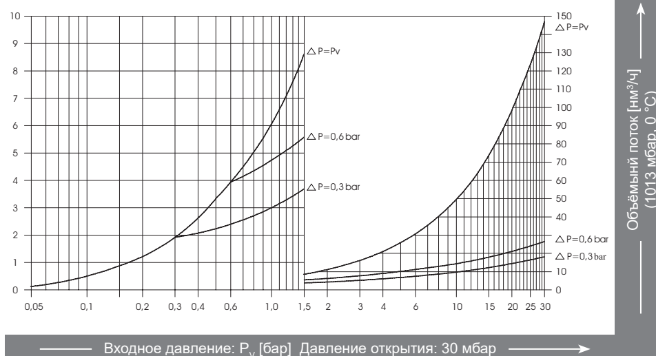
Диаграмма пропускной способности (воздух, 20 °C)
